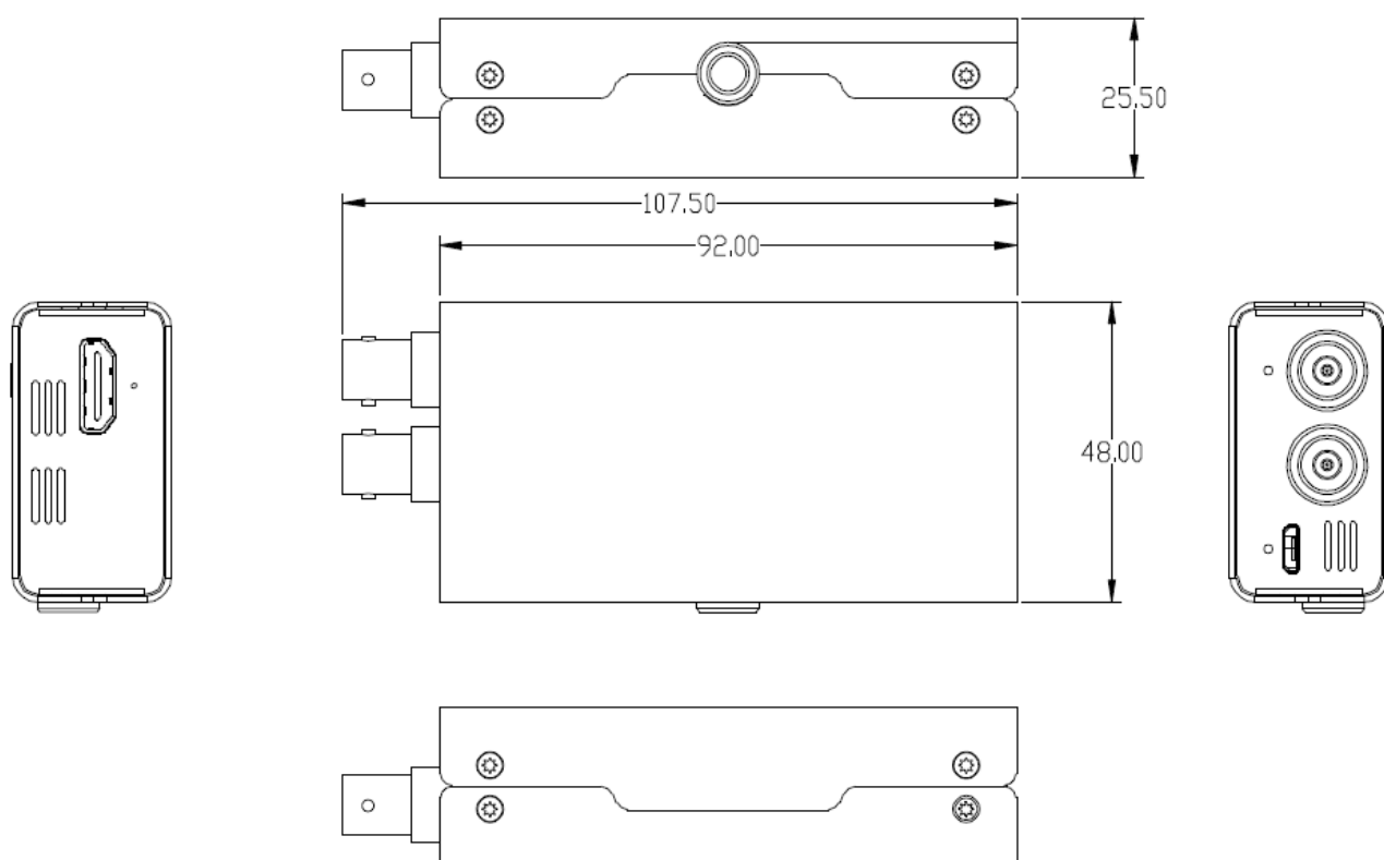
产品结构图
