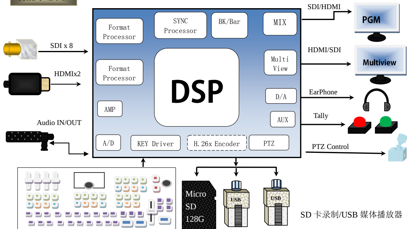
功能示意图
